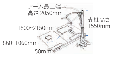
● B セット外観寸法
